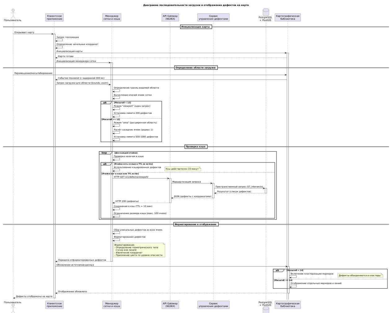
Рисунок 7 — Диаграмма последовательности загрузки и отображения дефектов
