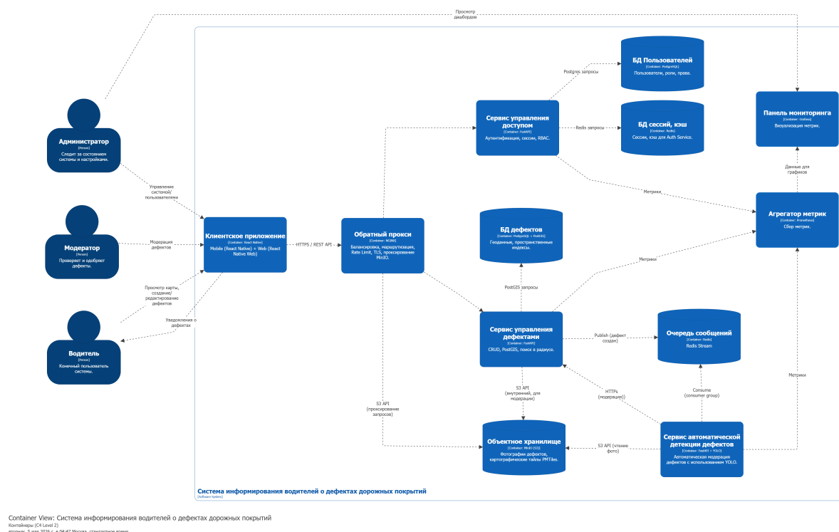
Рисунок 3 — Диаграмма контейнеров в нотации C4
