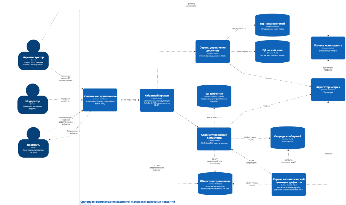
Рисунок 3 — Диаграмма контейнеров в нотации C4
