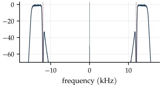
(d) output: \text{Re}\{ \cdot e^{j2\pi(f_c + f_0)t} \} , USB
