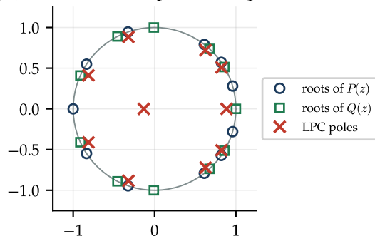
(d) Poles and line spectral frequencies
