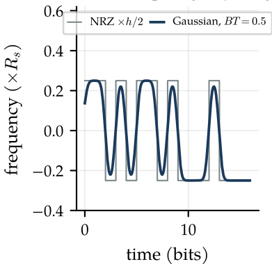
BLE 1M: frequency trajectory
