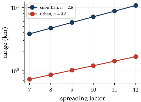
Range: 14 dBm, 10 dB fade margin
