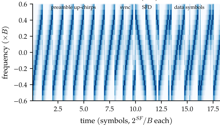
A LoRa frame (SF7)
