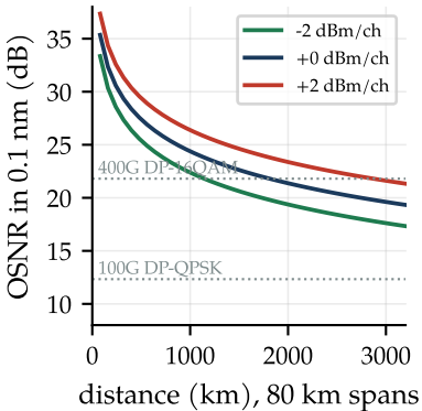
linear OSNR budget
