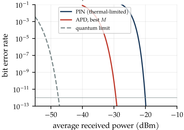
10 Gb/s OOK at 1550 nm
