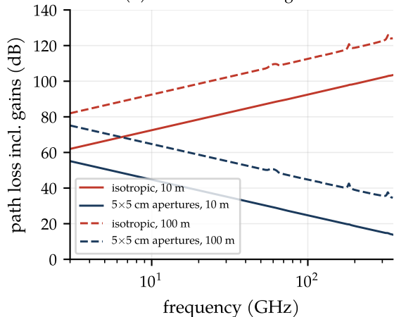
(b) the antenna-size argument
