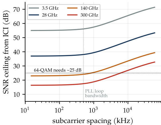
(b) phase-noise ICI after CPE removal
