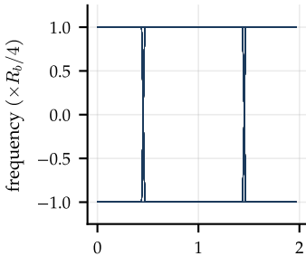
MSK
