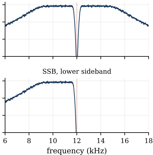
DSB-SC
