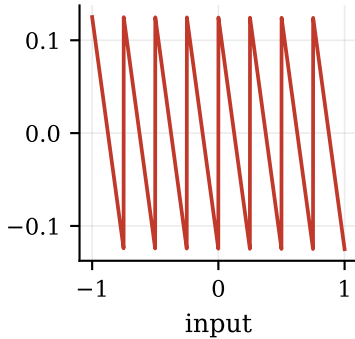
error e = Q(x) - x
