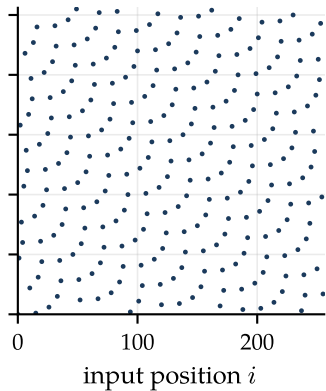
QPP (LTE), f_1=15 , f_2=32
