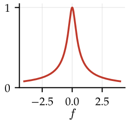
|Lorentzian|
