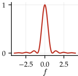
\text{sinc}^2
