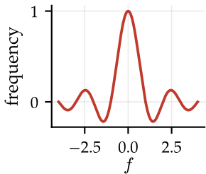
sinc
