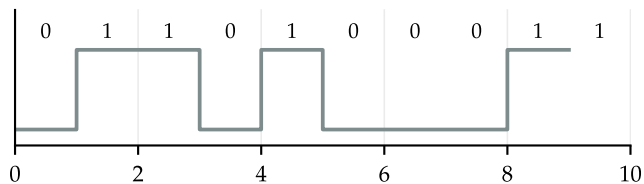
NRZ-L (polar)
