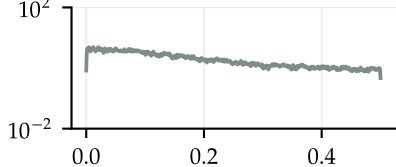
PSD S(f)
