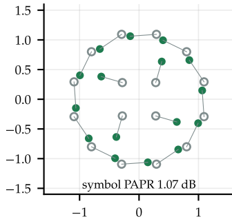
16-APSK (4+12)
