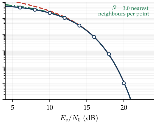
16-QAM
