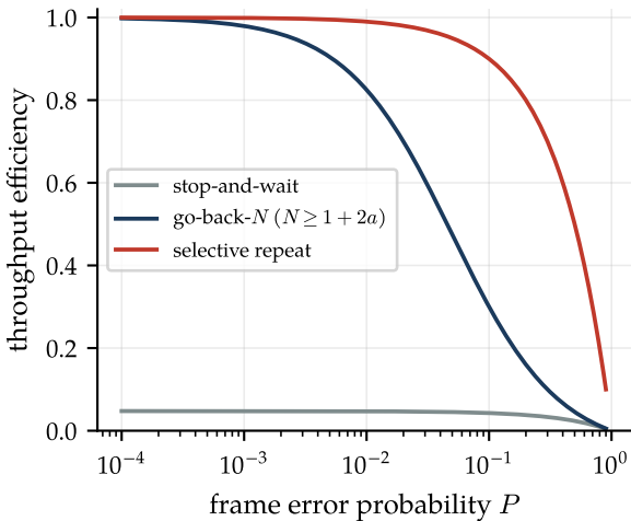
ARQ protocols, a = 10
