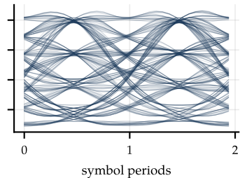
2 km, C band ( D=17 )
