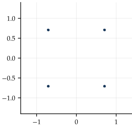
61-tap FIR: EVM -41 dB
