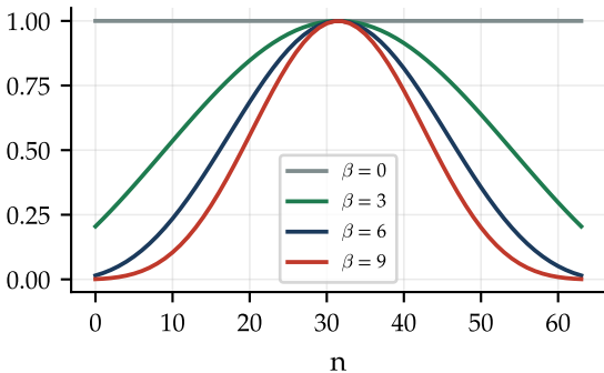
Kaiser windows, 64 points
