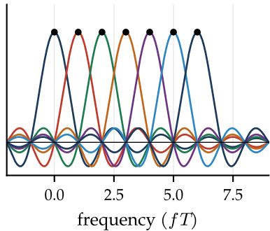
(c) OFDM: spacing 1/T
