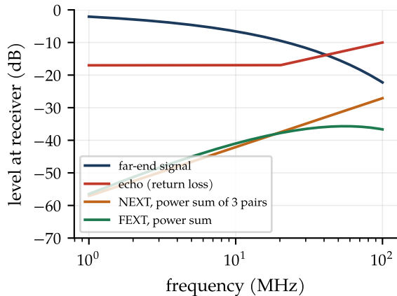
1000BASE-T: 100 m Cat 5e channel
