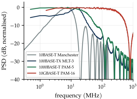
twisted-pair Ethernet spectra
