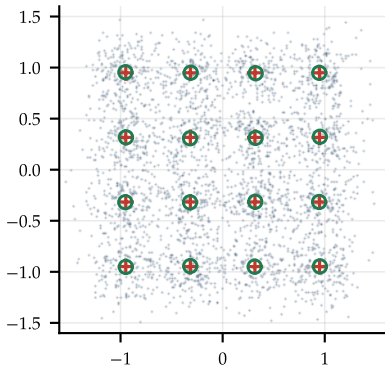
ZF SER = 1.2e-01
