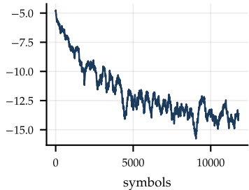
modulus error (|z|^2 - 1)^2
