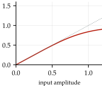
PA: compresses
