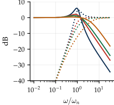
(c) |H| (solid), |1 - H| (dotted)
