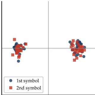
L-SIG: BPSK
