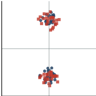
HT-SIG (11n): QBPSK
