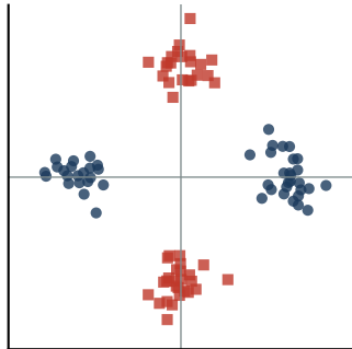
VHT-SIG-A: BPSK, then QBPSK
