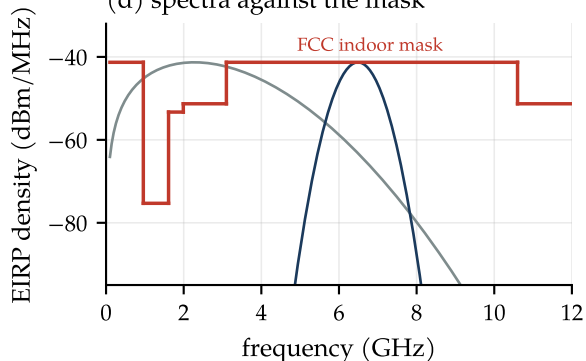
(d) spectra against the mask
