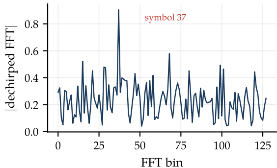
(d) spectra against the mask
