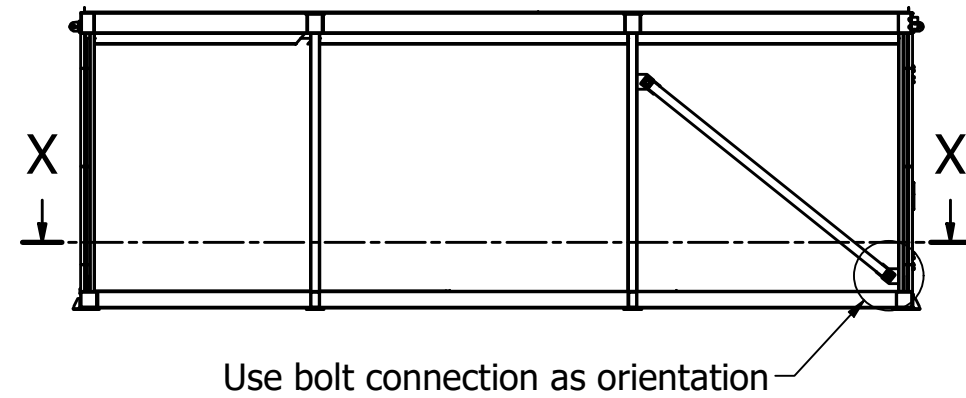
MV MODULE ( 1 : 100 )
