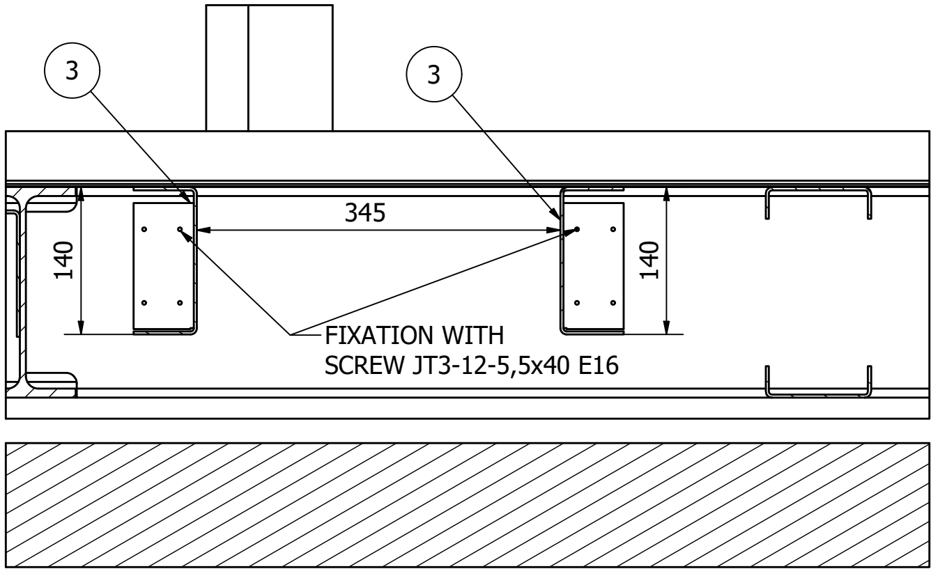
D-D ( 1:5 )
