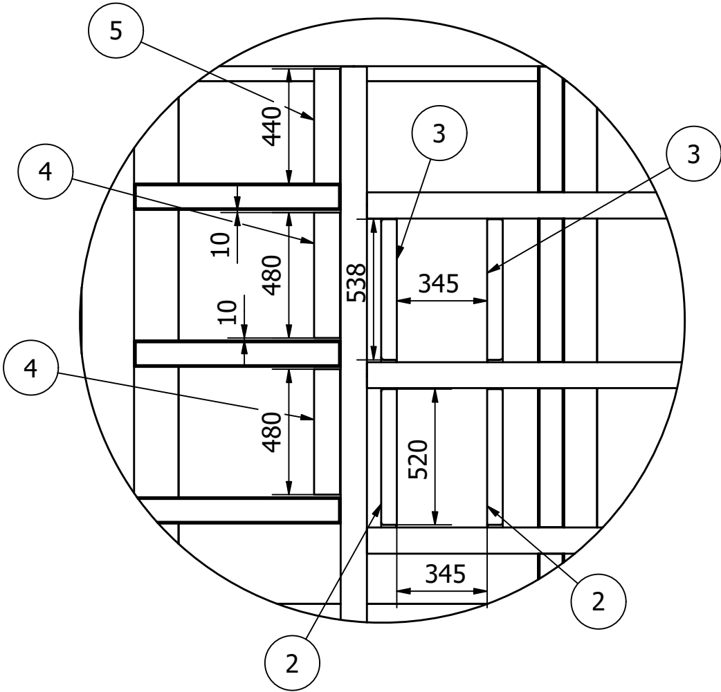
E ( 1:20 )
