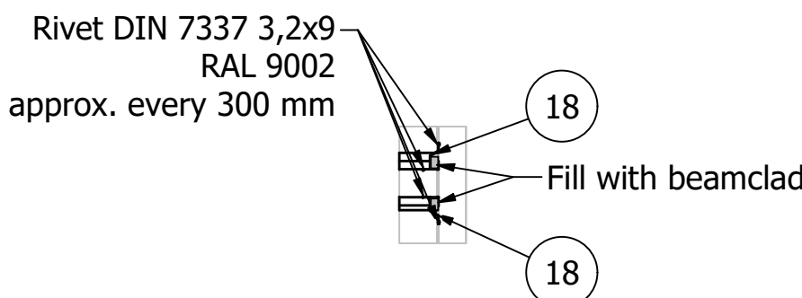
Y ( 1 : 25 )
