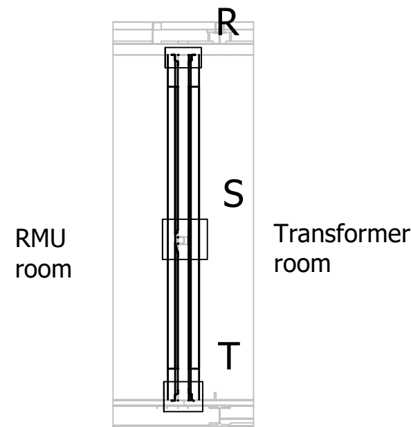
P-P ( 1 : 50 )
