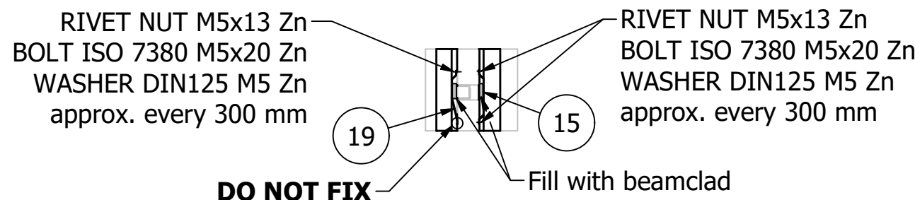
S ( 1 : 25 )
