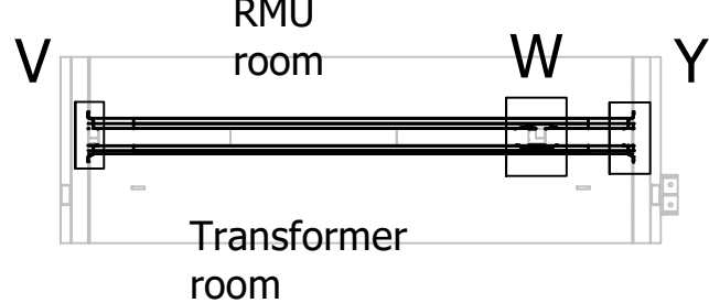
U-U ( 1 : 50 )
