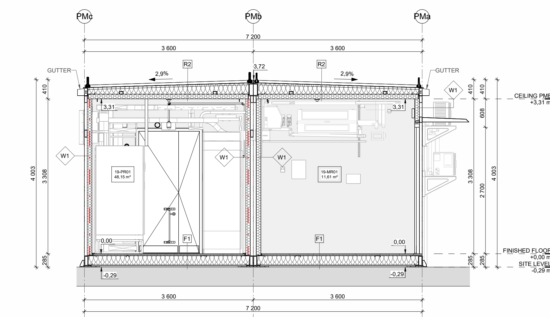
5 POWER MODULE - SECTION 1-1 1:50
