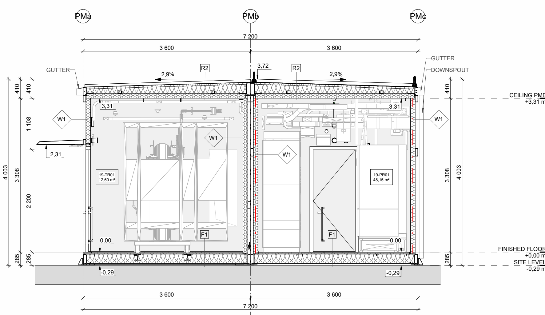
6 POWER MODULE - SECTION 2-2 1:50
