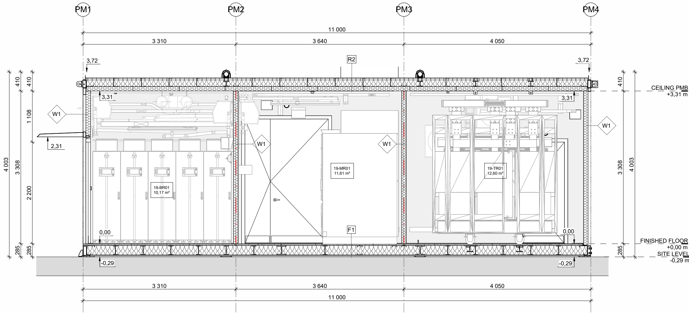
1 POWER MODULE - SECTION A-A 1:50
