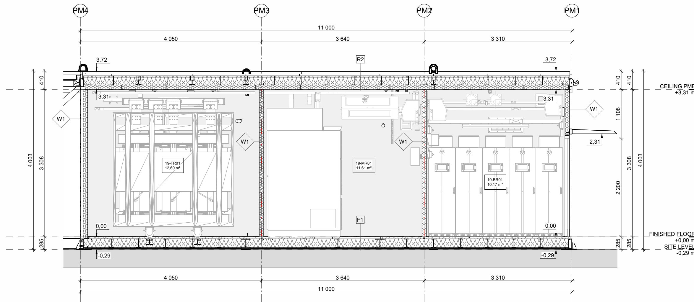
2 POWER MODULE - SECTION B-B 1:50
