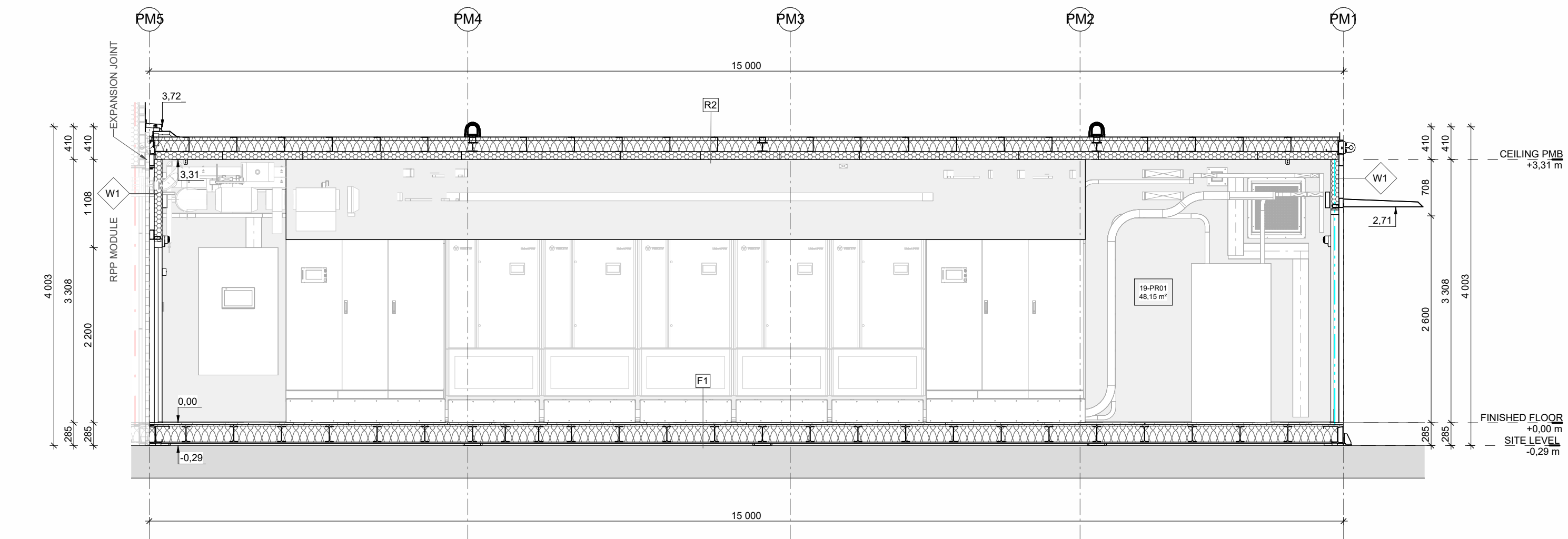
4 POWER MODULE - SECTION D-D 1:50
