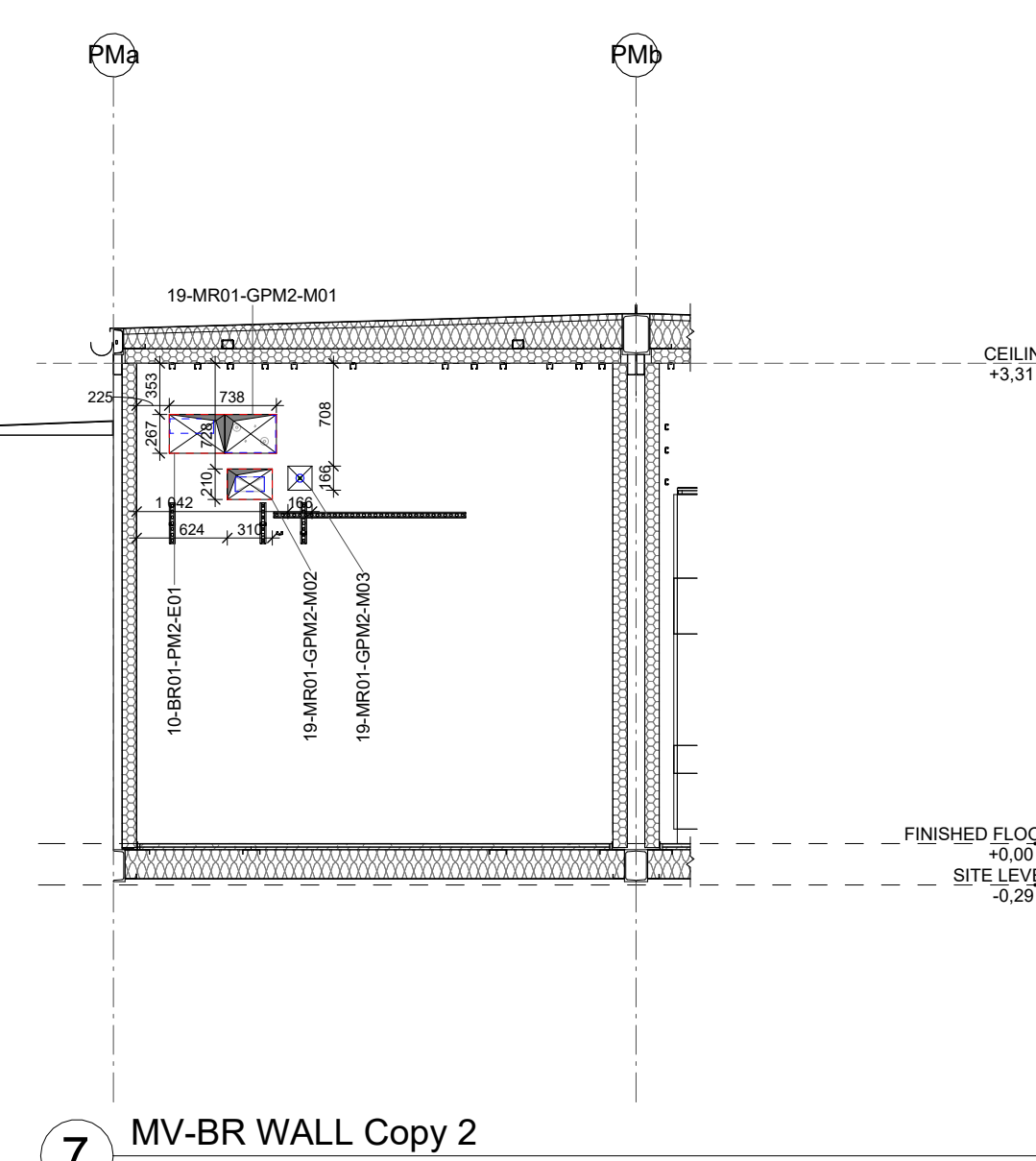
7 MV-BR WALL Copy 2 1 : 50
