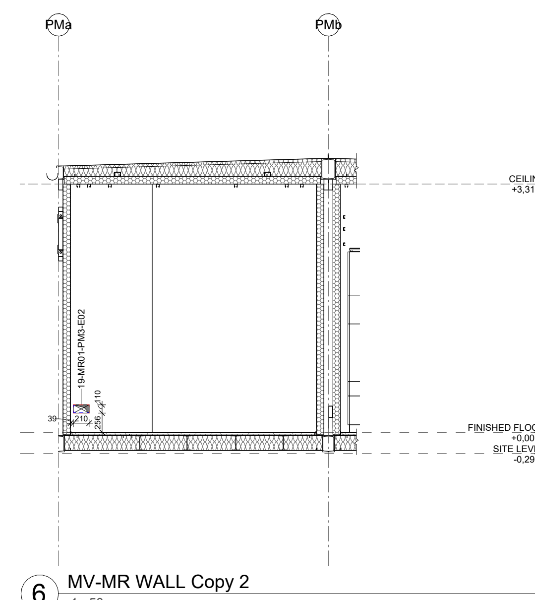
6 MV-MR WALL Copy 2 1 : 50
