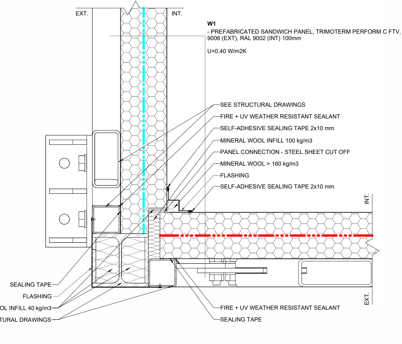
H09 PM/MS - MODULE CORNER 1:5
