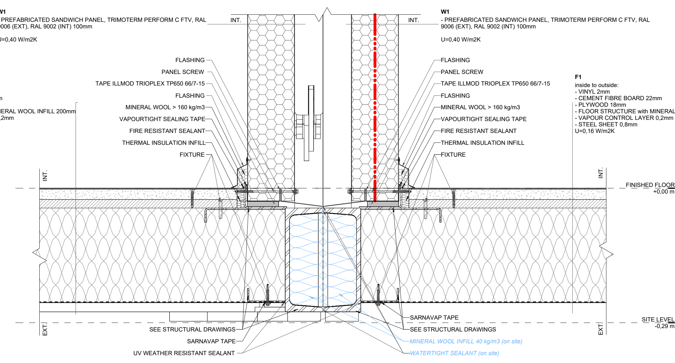
V08 PM/MV - MODULE CONNECTION-FLOOR 1:5
