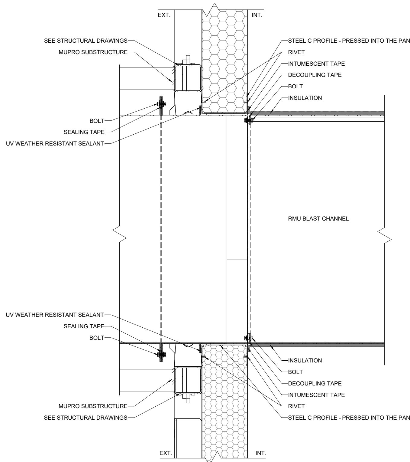
P13 RMU ARC BLAST 1:5
