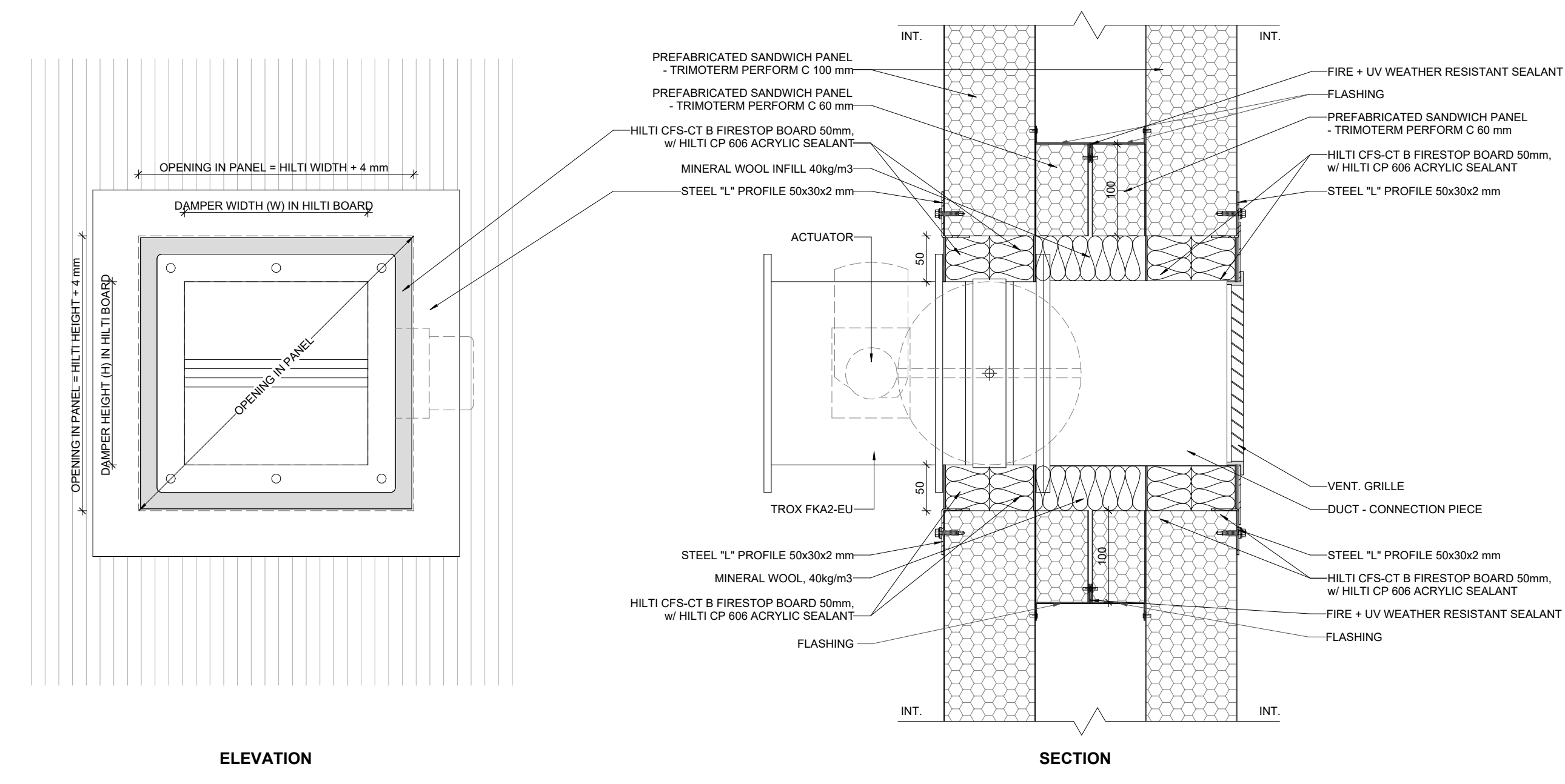
P08 TROX FKA2-EU 1:5
