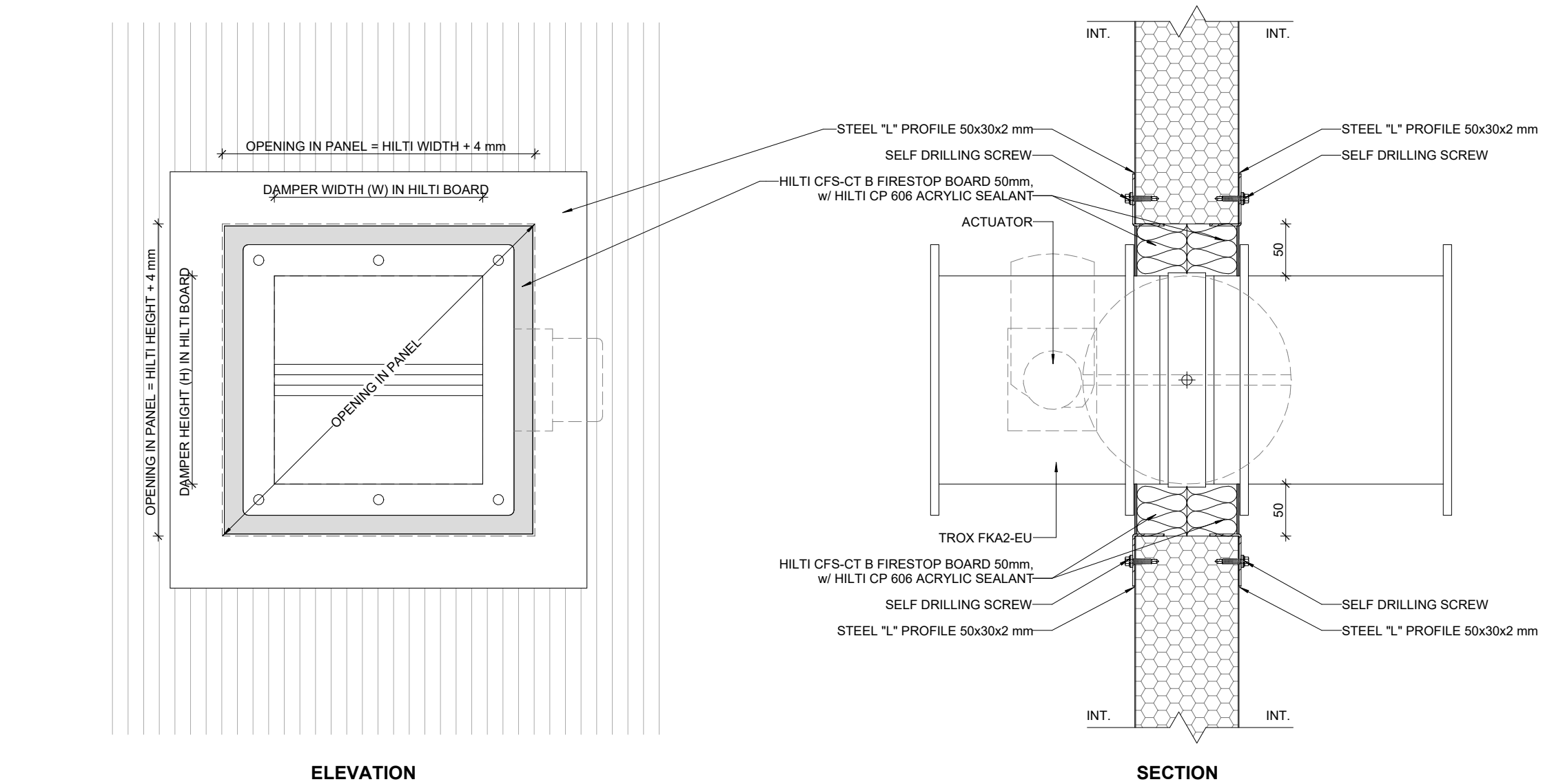
P07 TROX FKA2-EU 1:5
