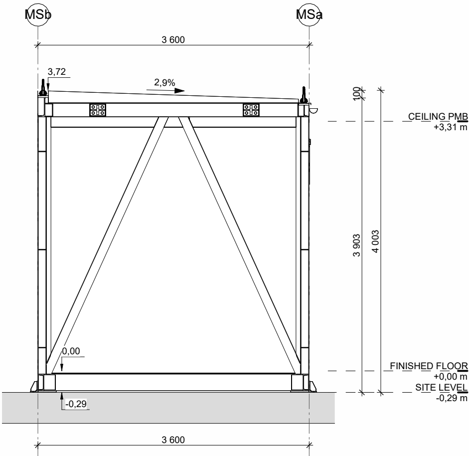
1 MS MODULE - ELEVATION EAST 1 : 50
