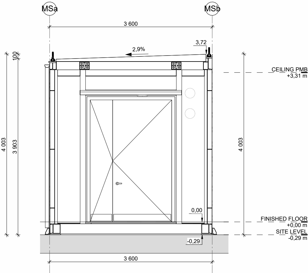
3 MS MODULE - ELEVATION WEST 1 : 50
