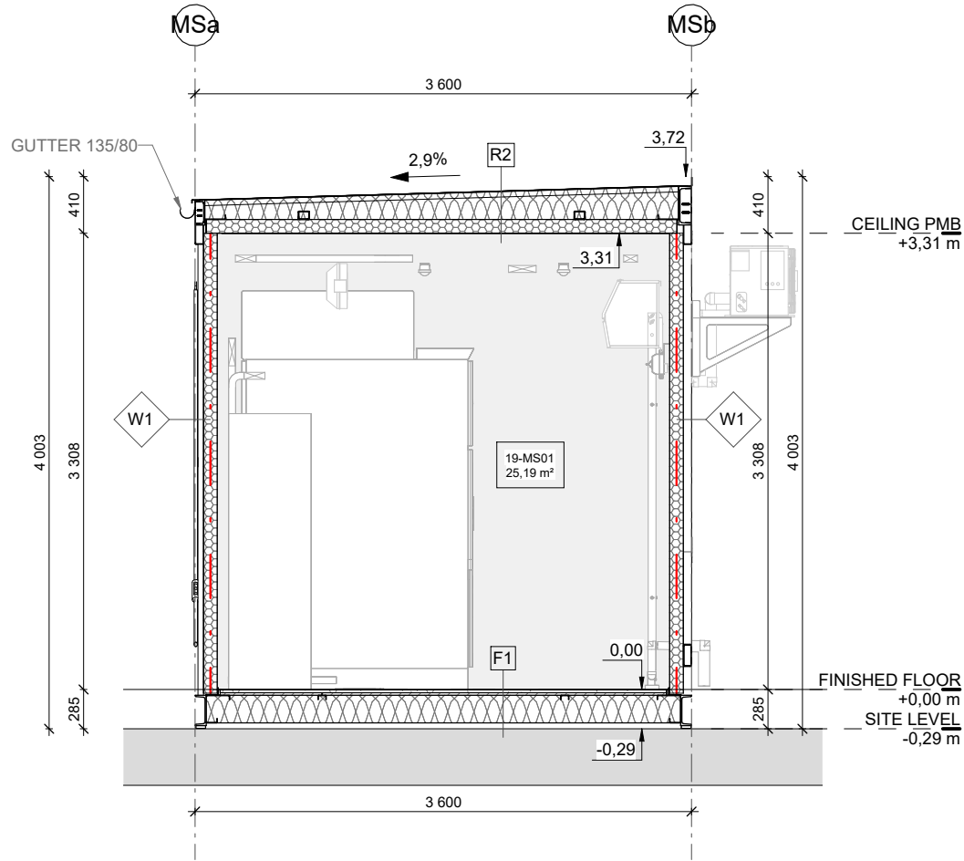
2 MS MODULE - SECTION 2-2 1 : 50
