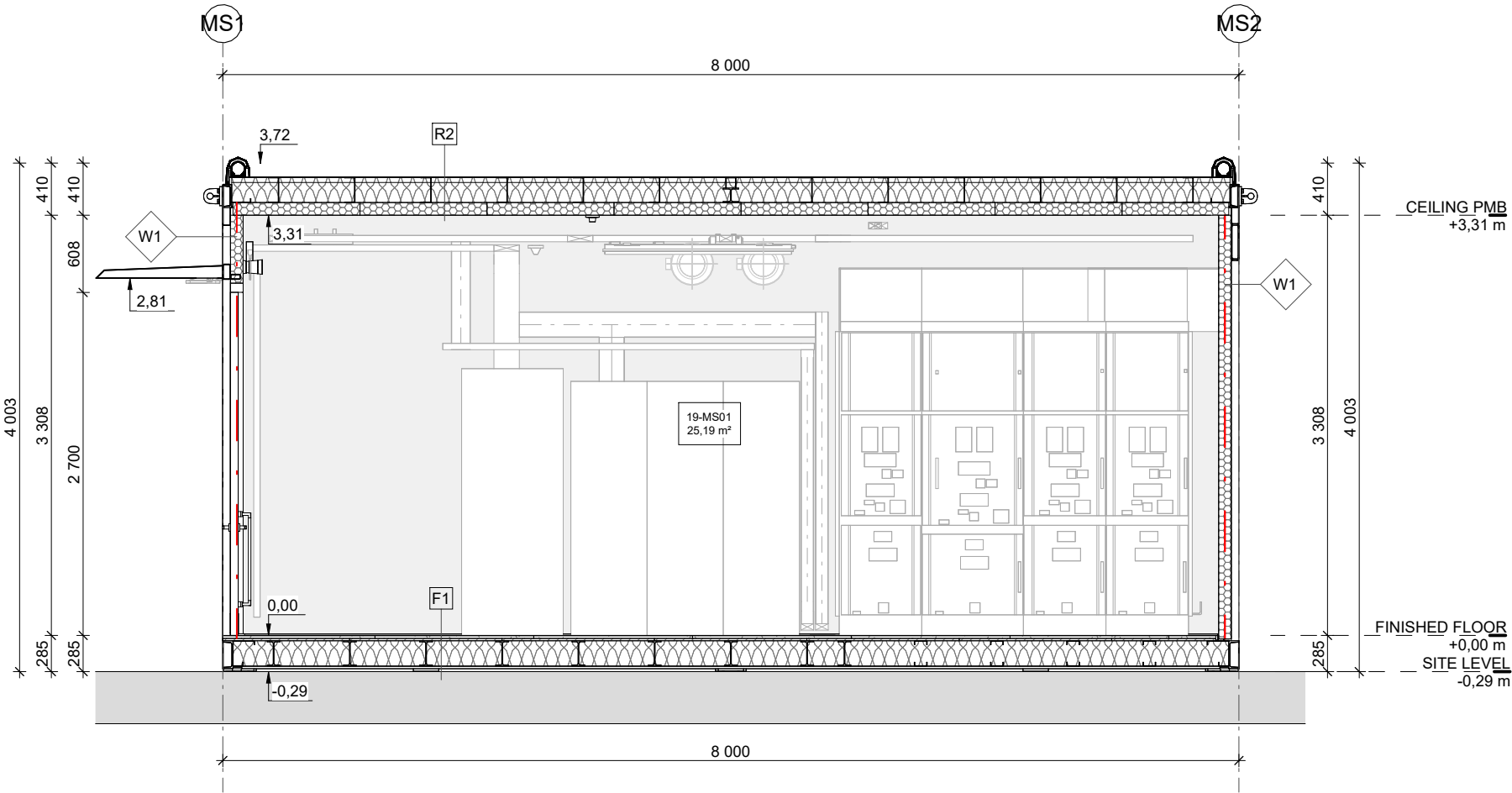
A MS MODULE - SECTION A-A 1 : 50
