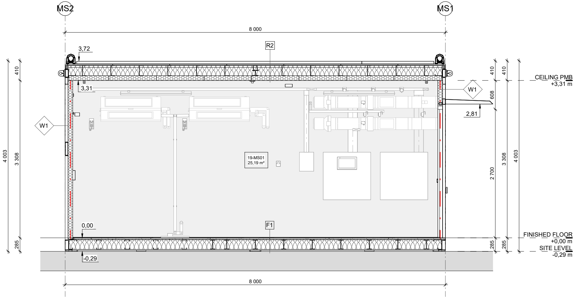
B MS MODULE - SECTION B-B 1 : 50
