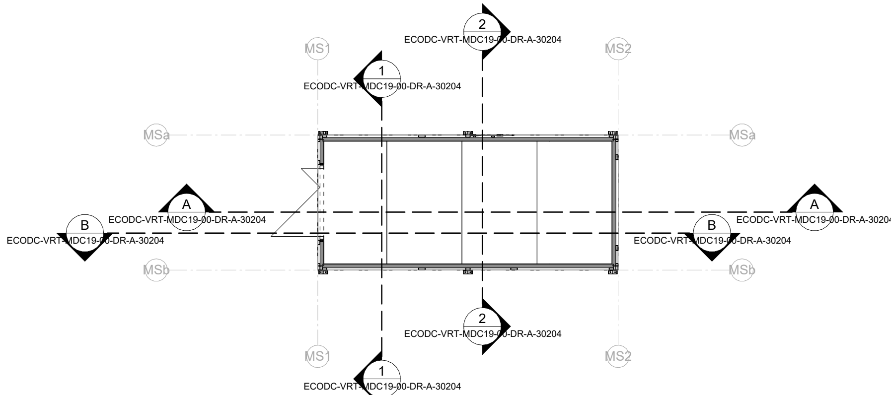
KEY PLAN - MS MODULE SECTION POSITIONS 1 : 100
