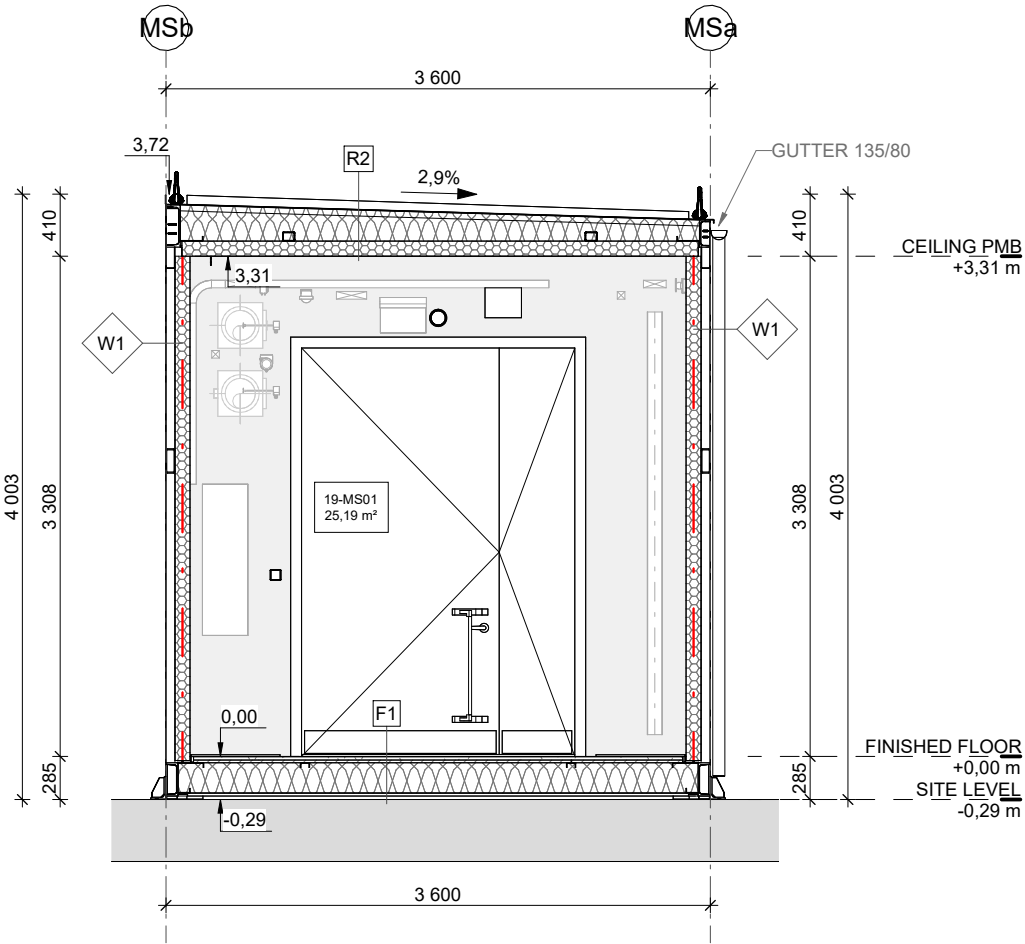
1 MS MODULE - SECTION 1-1 1 : 50
