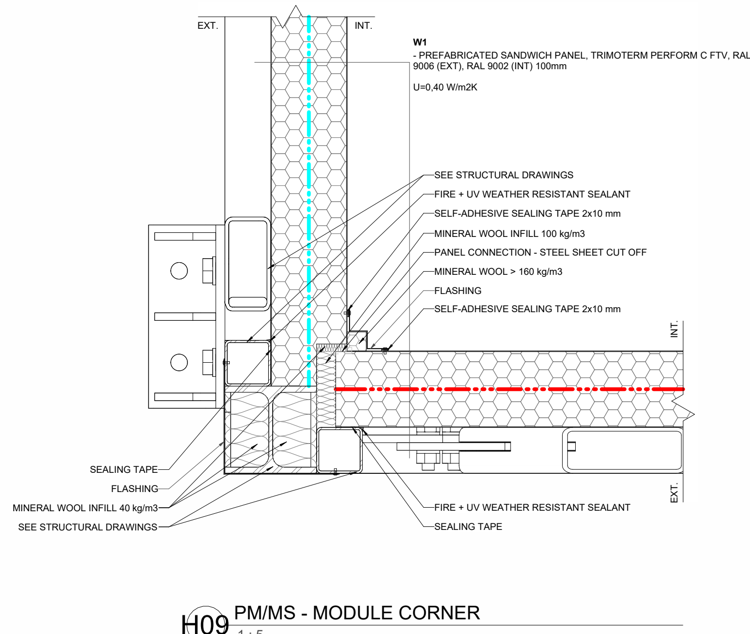
H09 PM/MS - MODULE CORNER 1:5
