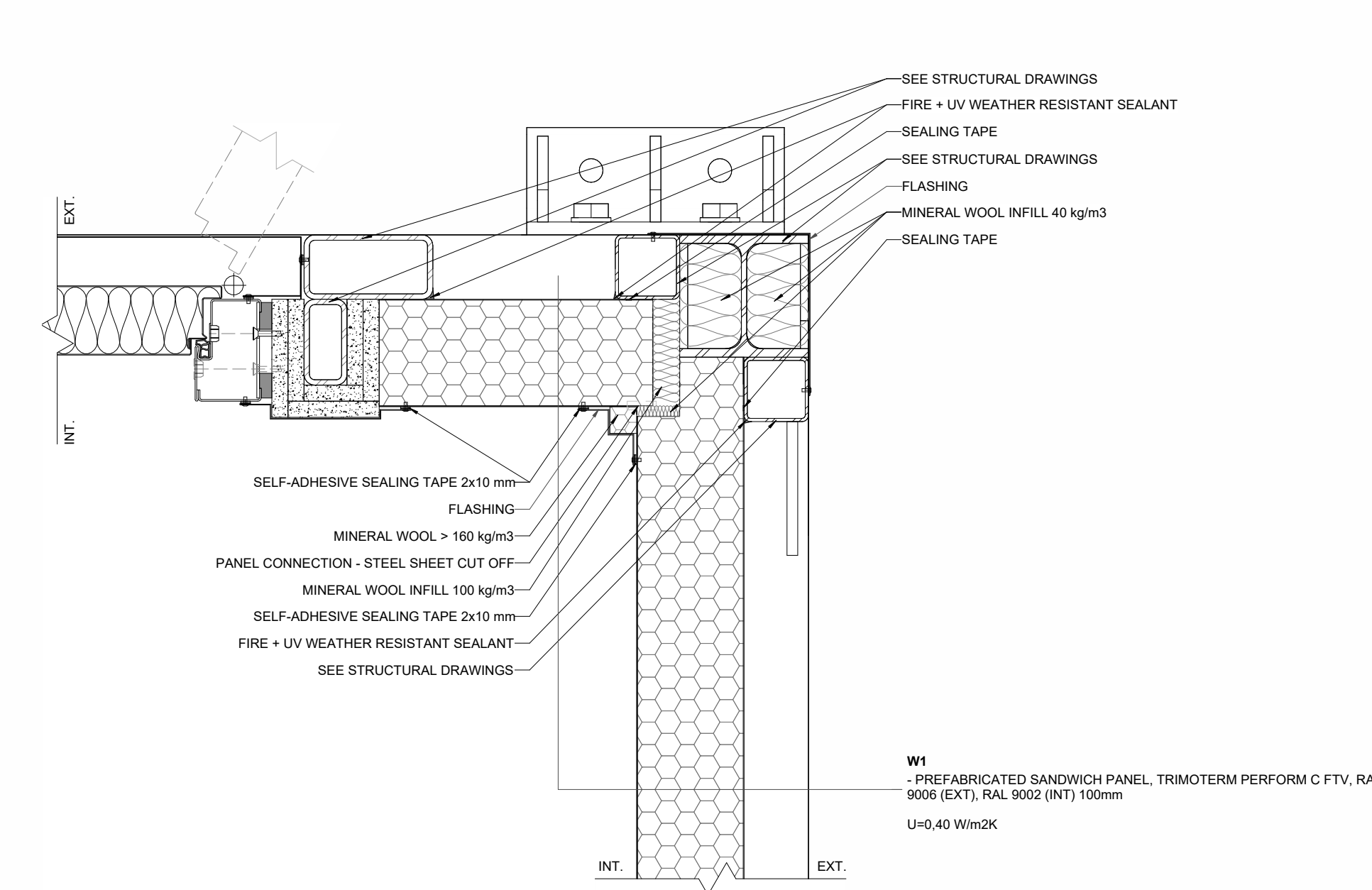
H04 MV - MODULE CORNER 1:5
