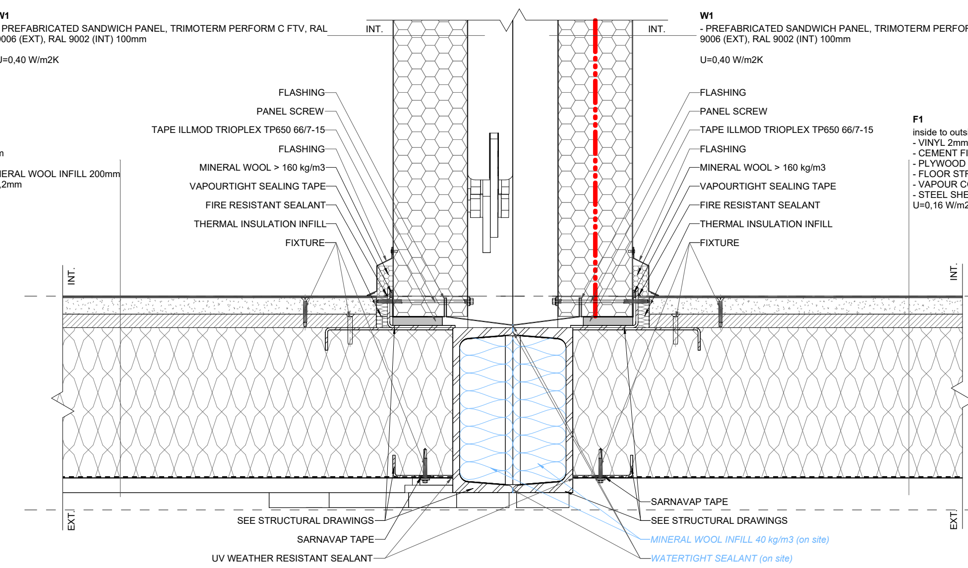
V08 PM/MV - MODULE CONNECTION-FLOOR 1:5
