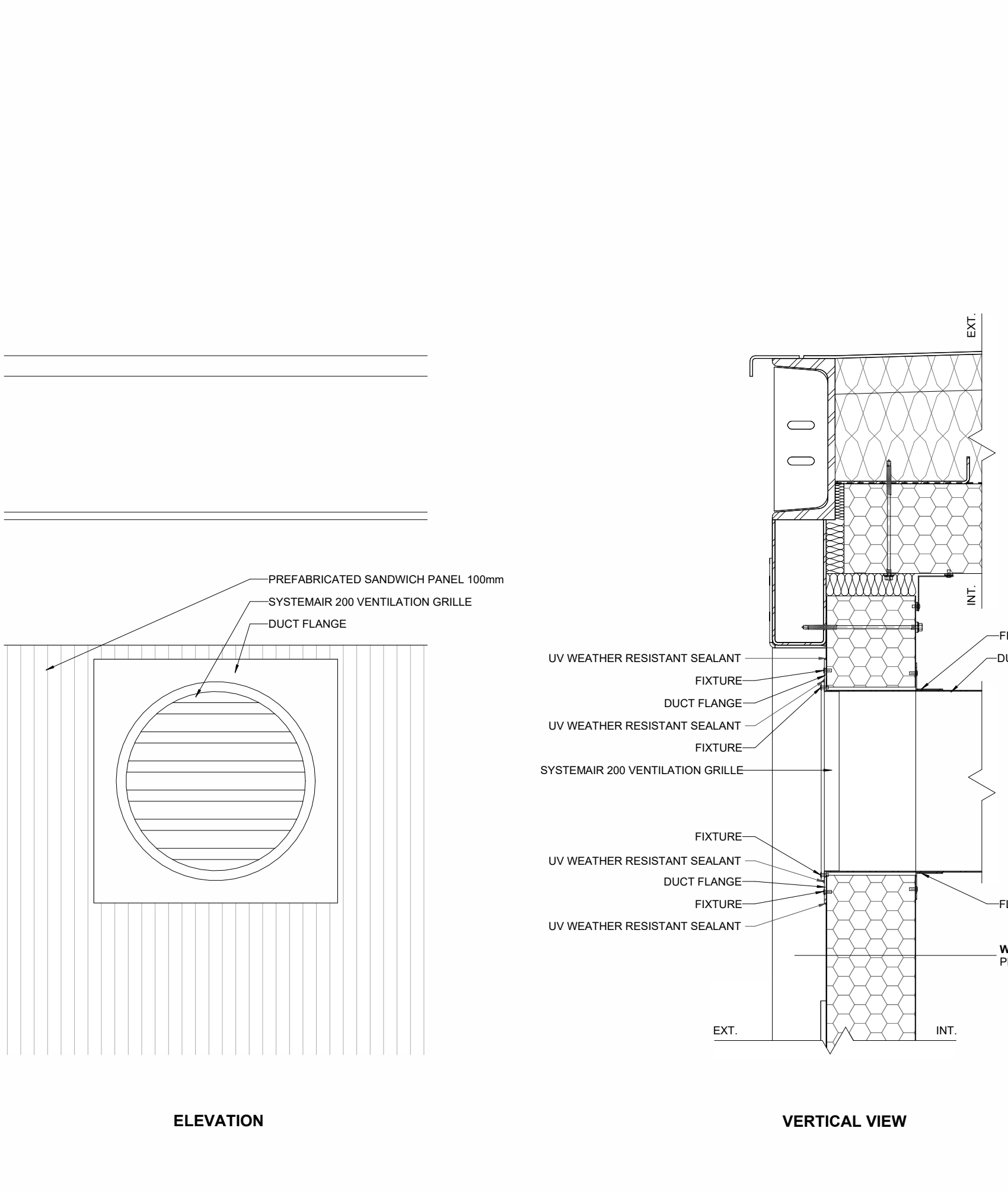
P16 SYSTEMAIR VENTILATION GRILLE 1:5
