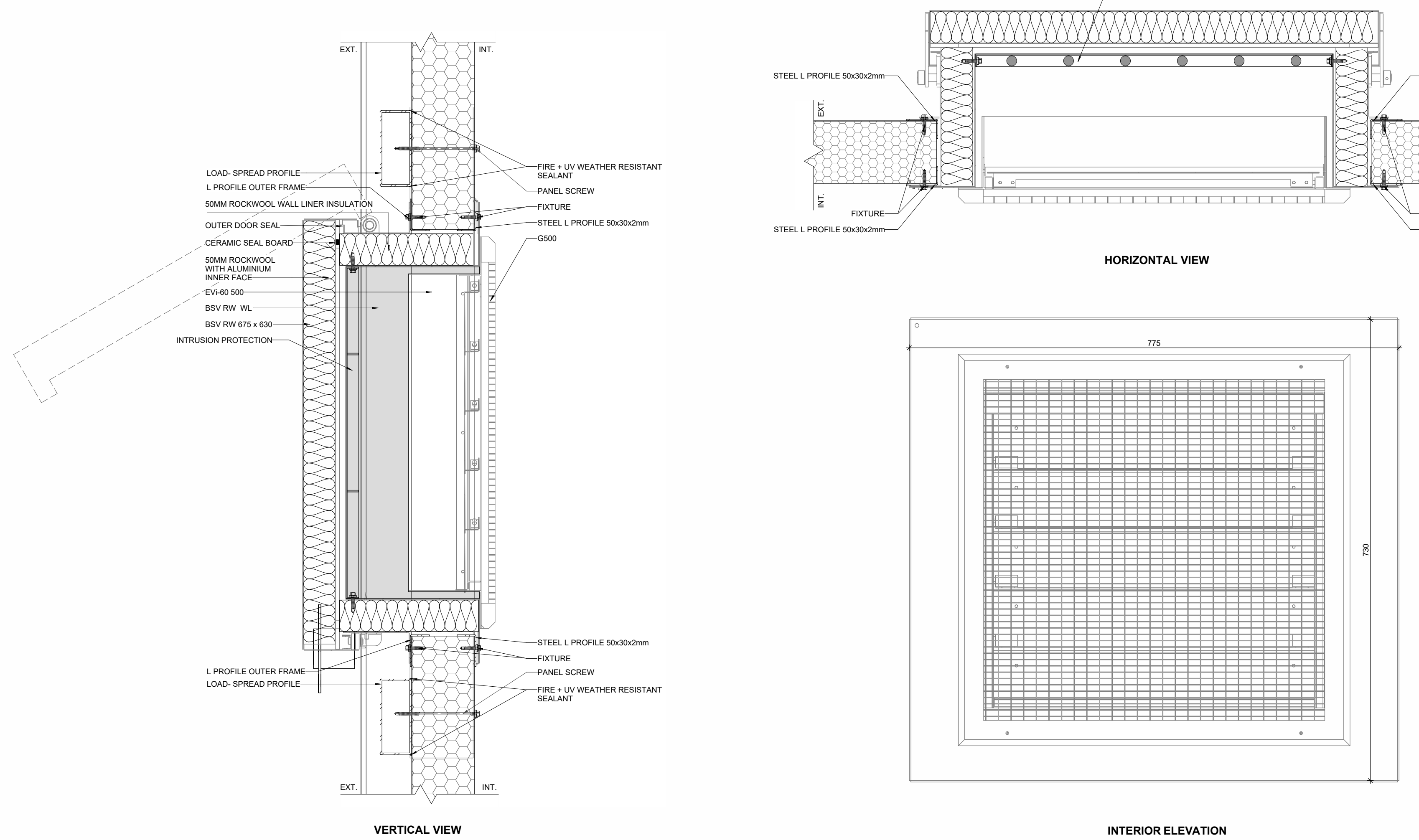
P10b BSV + EVI500 + SGHD 1:5
