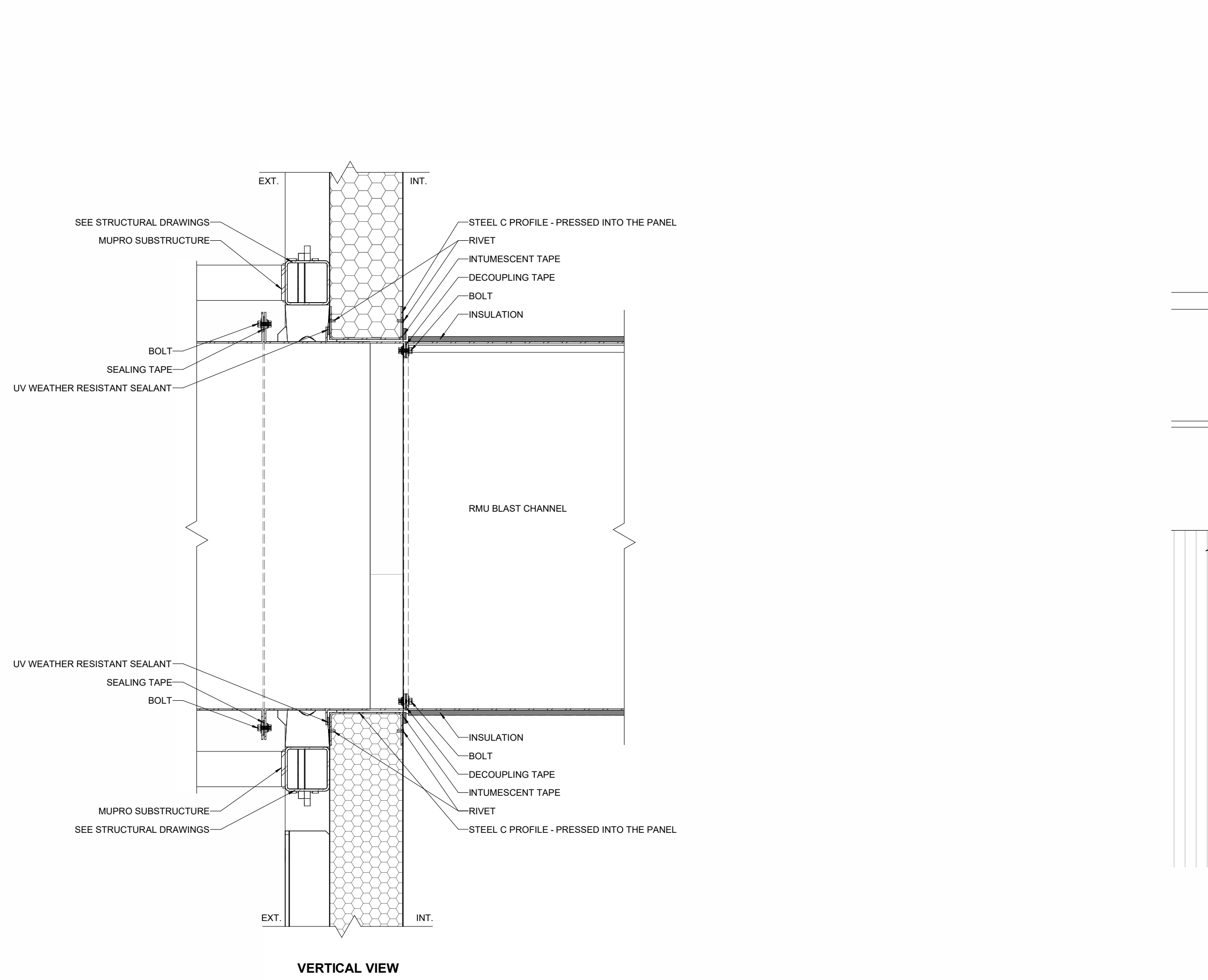
P13 RMU ARC BLAST 1:5
