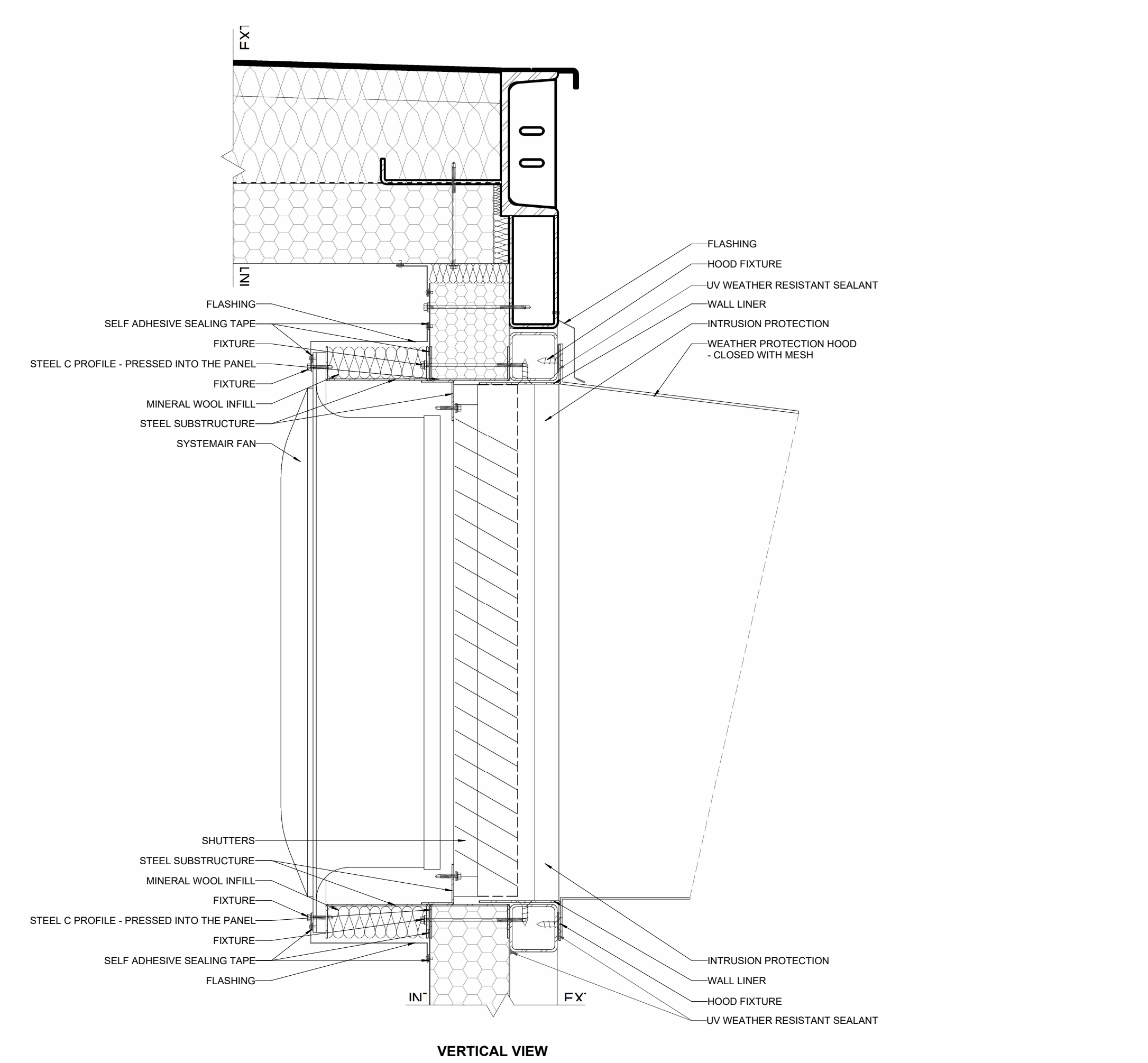
P12 SYSTEMAIR FAN 1:5
