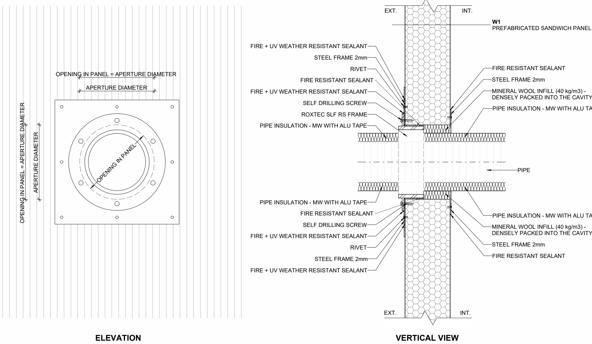
P02 ROXTEC SLF RS - EXTERIOR WALL 100 mm 1:5
