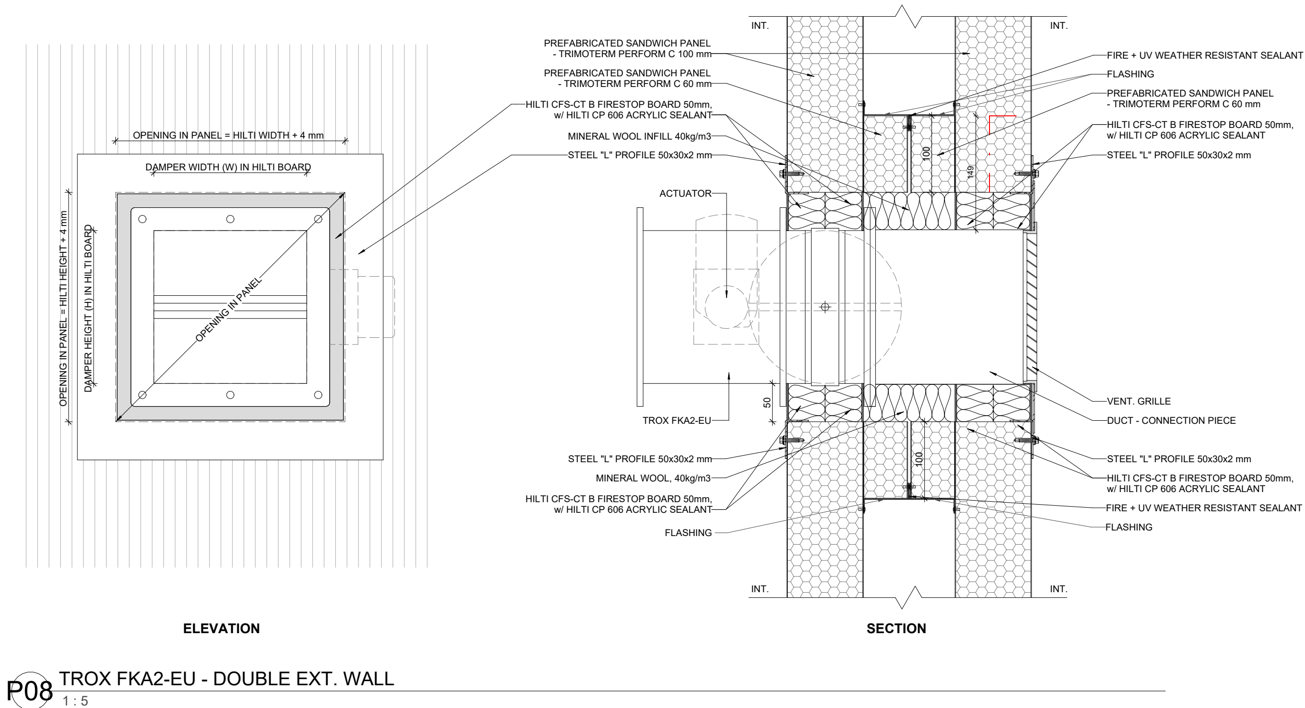
P08 TROX FKA2-EU - DOUBLE EXT. WALL 1:5
