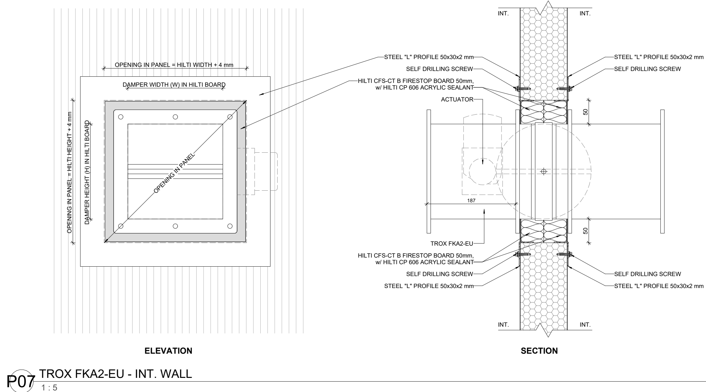
P07 TROX FKA2-EU - INT. WALL 1:5
