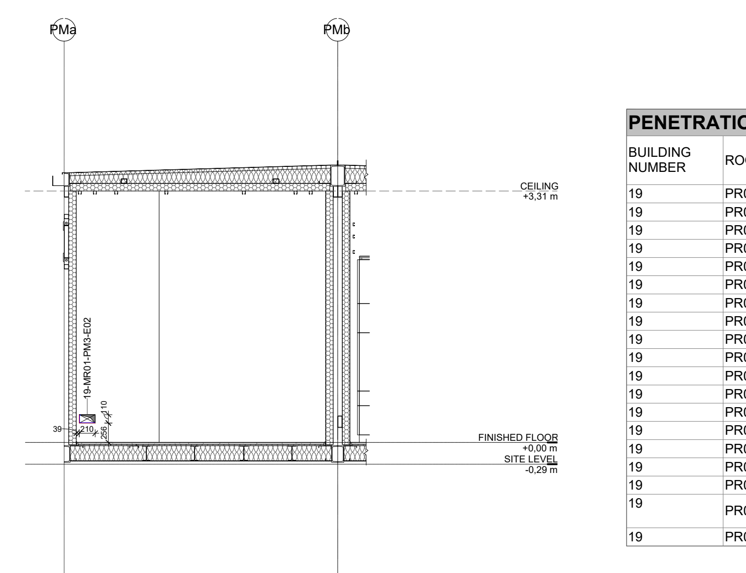
6 MV-MR WALL 1:50
