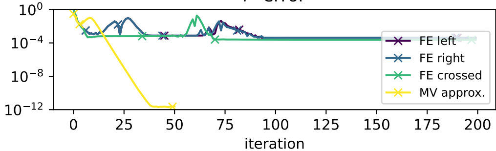
l^2 error
