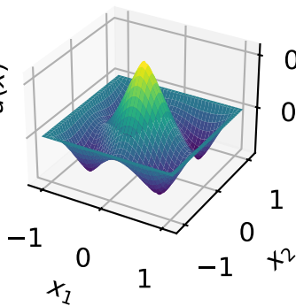
local extremum
