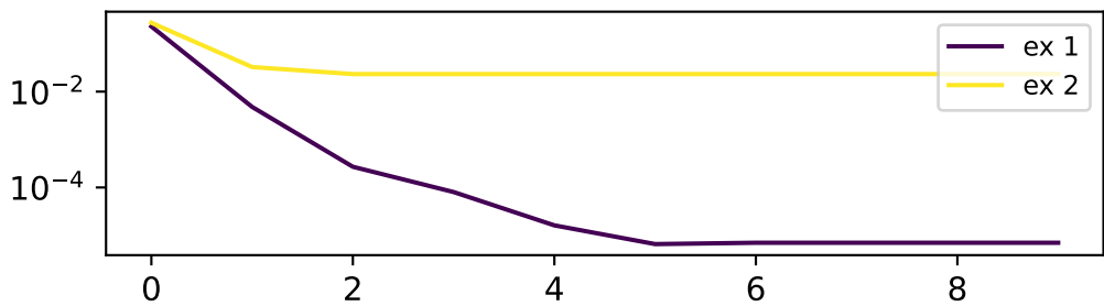
l^2 error
