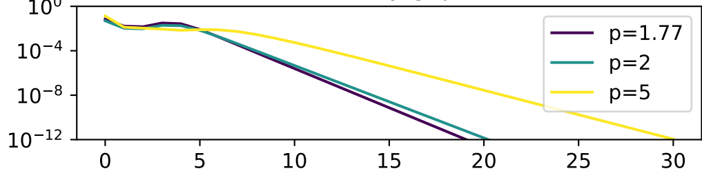
l^2 error
