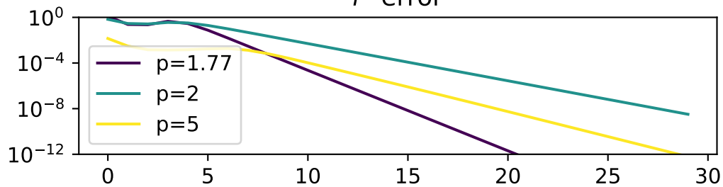
l^2 error
