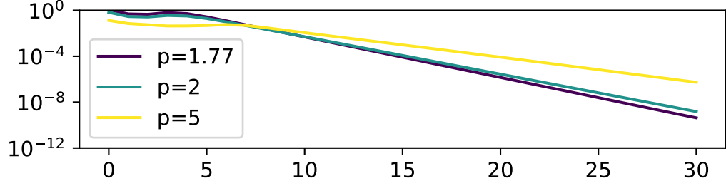
l^2 error
