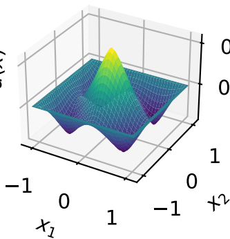
local extremum
