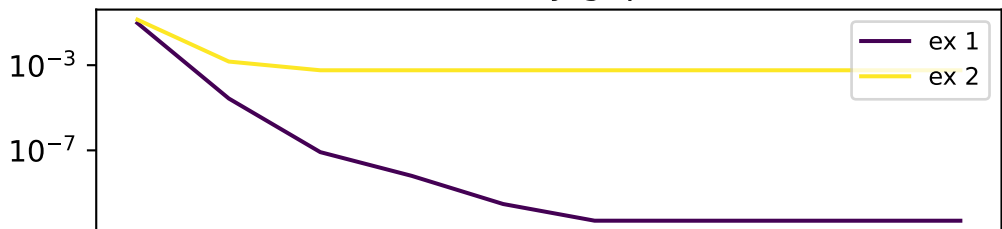
l^2 error
